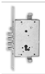
FIAM 672 GF (ISEO)
